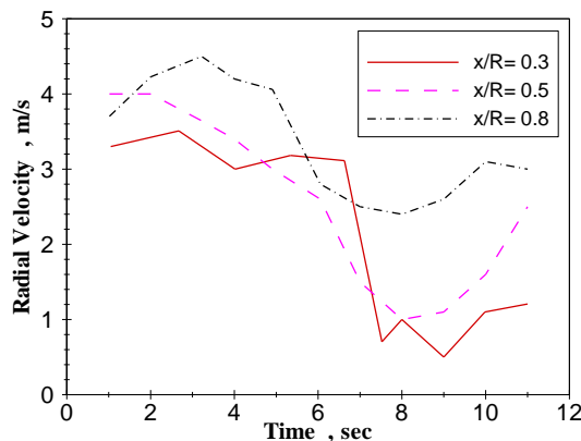
شکل ۱- تغییرات سرعت شعاعی نسبت به زمان (B Nazanin ۱۰ pt, Bold)
